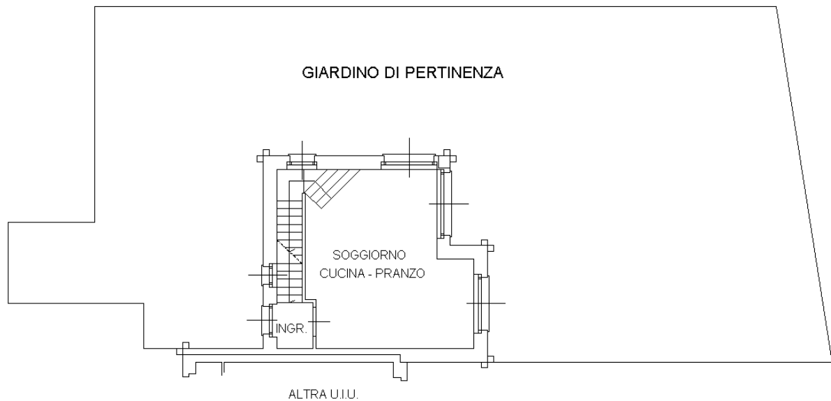
PIANTA PIANO TERRA H.2.70 MT.
