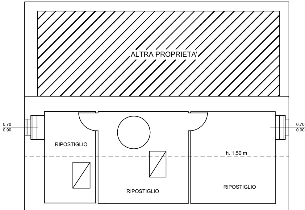
PIANO SECONDO (mansarda)
