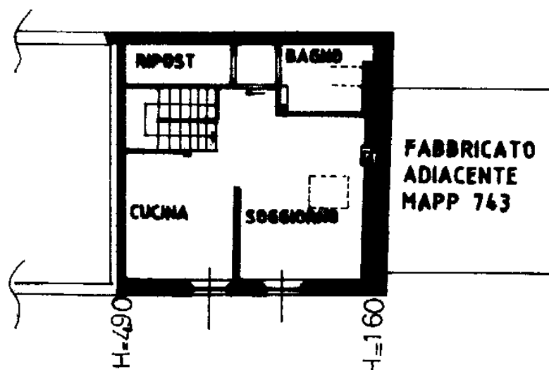
PIANO SECONDO / MANSARDA
