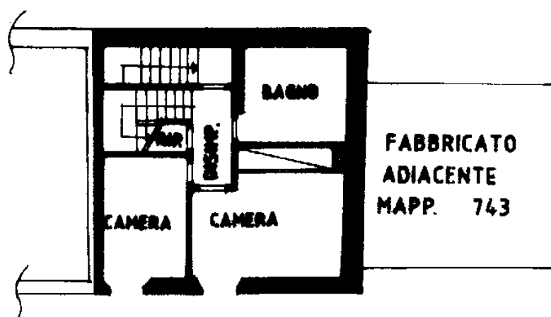
PIANO PRIMO H=2.45
