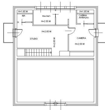
PIANTA PIANO SECONDO SOPPALCO
