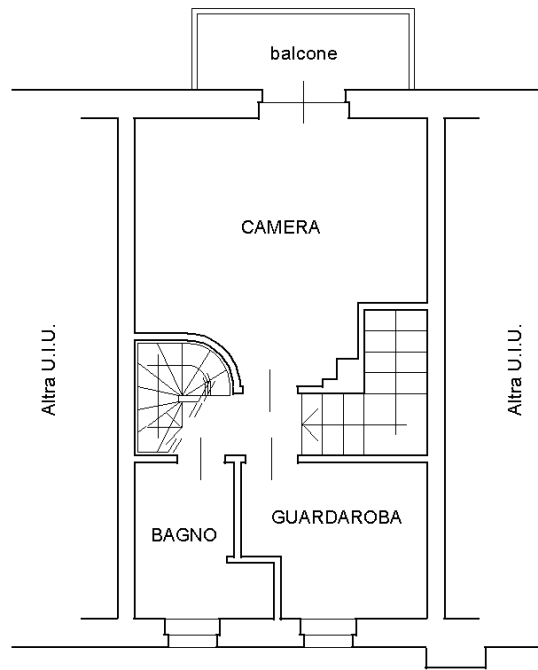
PIANO PRIMO H = ml. 2,40
