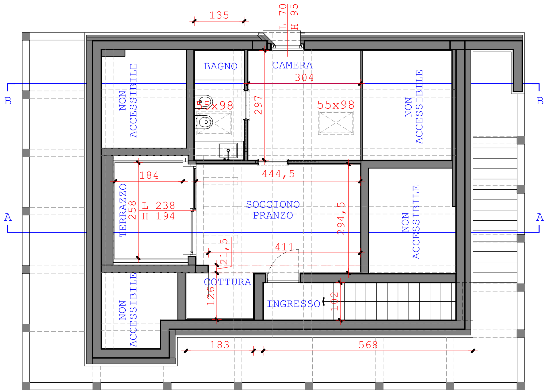
PIANTA PIANO SOTTOTETTO
