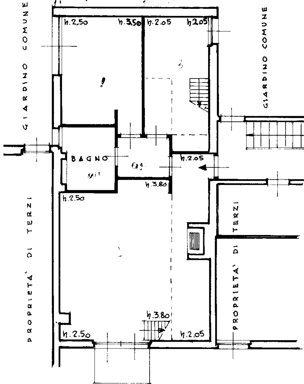
PIANO SECONDO
